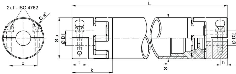
Distanzkupplung EWLH
