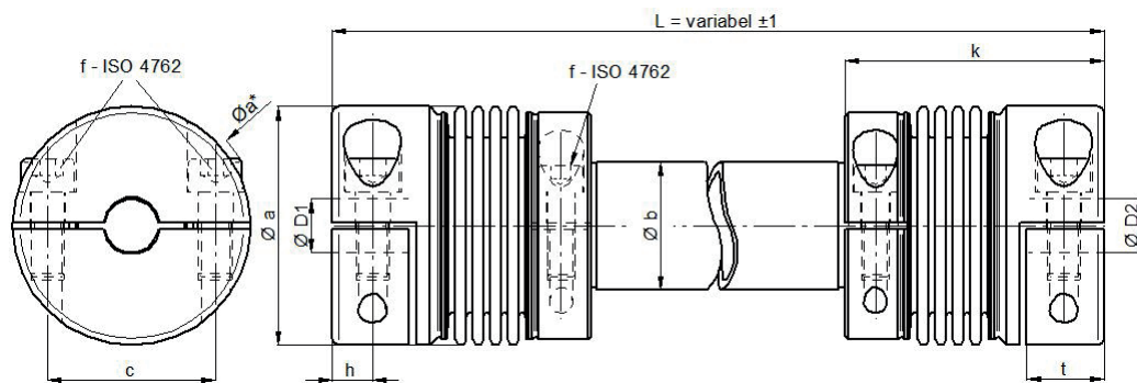
Distanzkupplung EWLC
