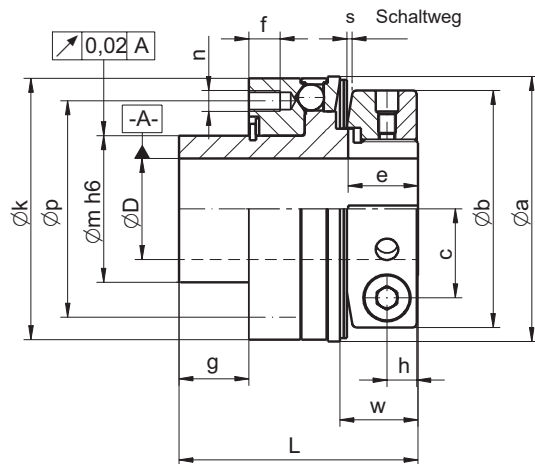
Sicherheitskupplung ECOL
