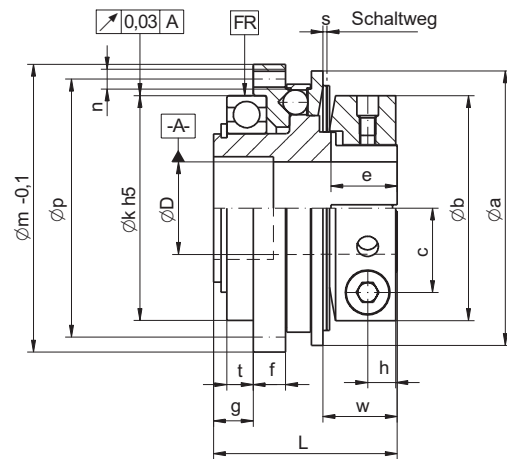
Sicherheitskupplung ECP
