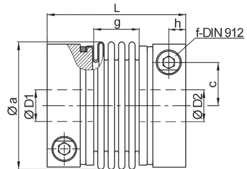
Metallbalgkupplung EWB
