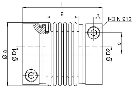
Metallbalgkupplung EWA
