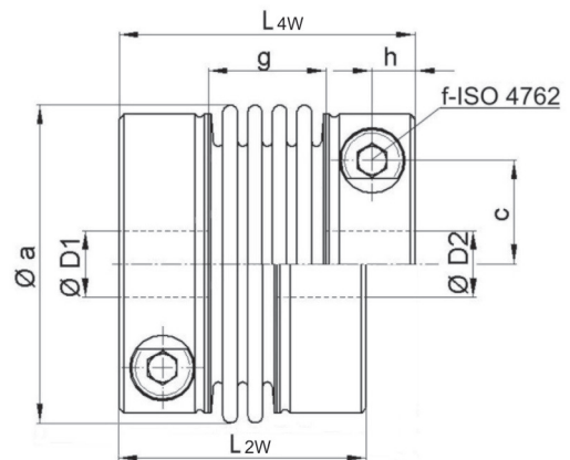
Metallbalgkupplung EWF
