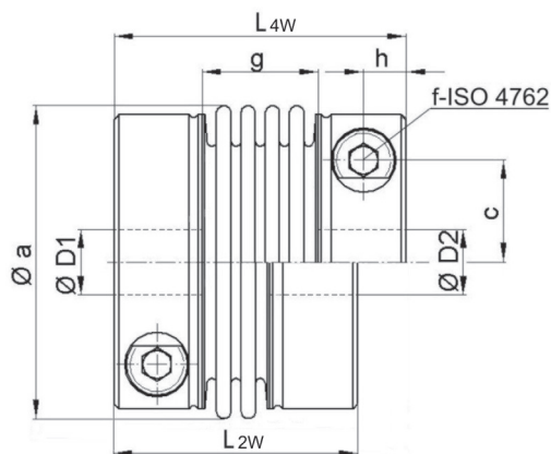
Metallbalgkupplung EWC
