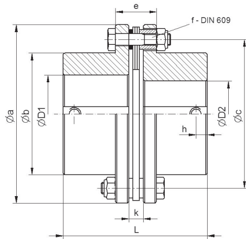
Lamellenkupplung EWZK
