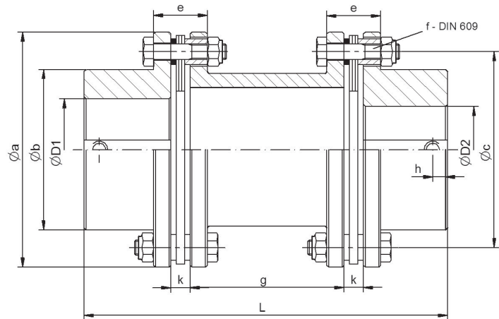
Lamellenkupplung EWZL
